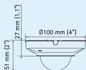
AXIS M3004-V AXIS M3005-V
