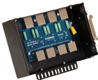
Názorná ukázka montáže modulů do krytu
